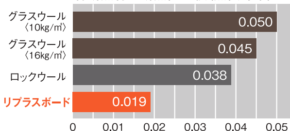
各断熱材の断熱性比較(熱伝導率)
