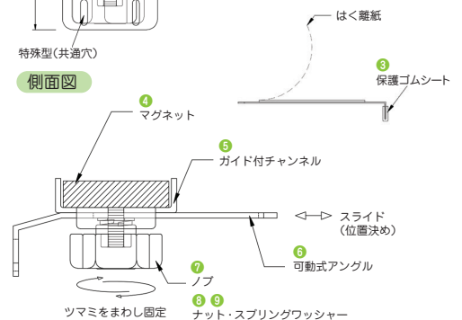
チラシブロックエントランス用標準型 (OCB-ST01-12)
